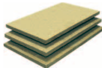
Каменно-минерална вата Fibran Geo Размери: 1000x600x50 мм За звуко-и топлоизол. Плътност: 30 кг/м 3 Топлопроводимост: 0,034 W/mK 7,2 м 2 /пакет, продажба на пакет 21.53 хх 21955105
