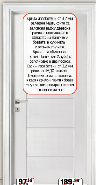
Интериорна врата Троя, грундирана с каса 7 см Размери: 70/80/90x200 см дясна/лява Код: 03801413/ 03801420/ 03801635 03801642/ 03801659/ 03801666
