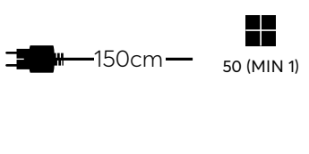
SET FOR 2-WAY ROPELIGHT 1,5M, PLUG, MAX CONNECT 50M, 1 PC PLUG 2WIRE WITH PIN + 1 MID-CONNECT 2W PIN+ 13MM END CAP + 2 HEAT SHRINKABLE TUBES + 1 GLUE ΣΕΤ ΓΙΑ ΜΟΝΟΚΑΝΑΛΗ ΦΩΤΟΣΩΛΗΝΑ, 1,5Μ, ΦΙΣ, MAX ΣΥΝΔΕΣΗ 50Μ, 1 ΤΜΧ ΦΙΣ 2WIRE ΜΕ PIN + 1 ΣΥΝΔΕΣΗ 2W PIN + 13ΜΜ ΤΕΛΙΚΟ ΚΑΠΑΚΙ + 2 ΘΕΡΜΟΣΥΣΤΕΛΛΟΜΕΝΟΙ ΣΩΛΗΝΕΣ + 1 ΚΟΛΛΑ
